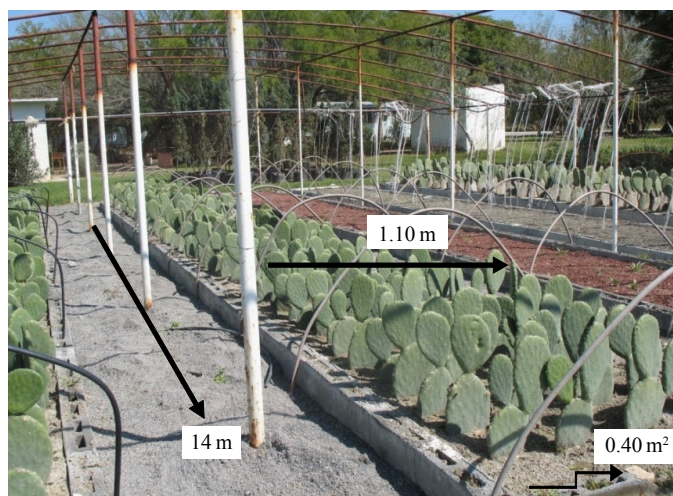
Figura 1. Sistema hidropónico cerrado de nopal con tres bancales de hormigón a cielo abierto.
