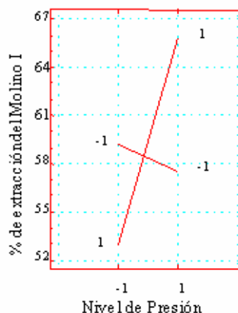
Figura 3 Interacción entre la Velocidad de la Picadora I y la Presión Hidráulica sobre el % de extracción del Molino 1.
