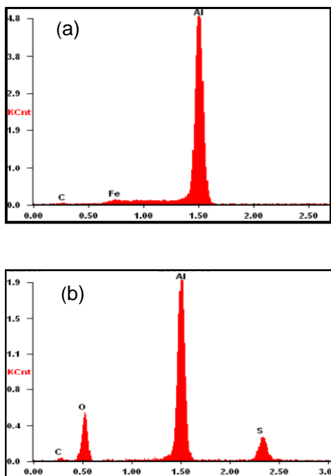
Figura 3. a) Imagen EDAX para el sustrato de aluminio. b) imagen EDAX para la lámina anodizada durante 1 hora en una solución al 20% de H_2SO_4 .
