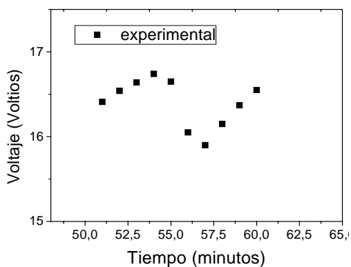
Figura 6. Formación de la zona II, que corresponde a la tipo porosa.
