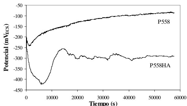
Figura 5. Variación del potencial de corrosión con el tiempo de inmersión en solución Ringer a 37 °C hasta 15 horas, para el acero Böhler P558 con y sin recubrimiento de hidroxiapatita.
