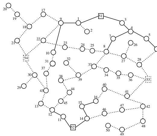
Figura 4. Planeamiento estático sistema de prueba 50 nodos.
