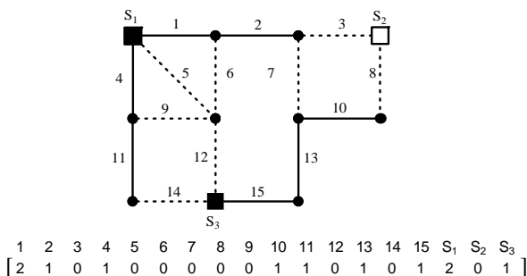
Figura 2. Representación del sistema de distribución.
