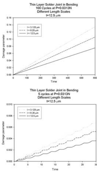
Figura 4. Soluciones mediante la teoriza de Cosserat para diferentes parámetros de escala en una microviga de 12.5\mu m .
