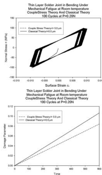
Figura 6. Soluciones mediante la teoriza de Cosserat y la clásica con igual carga para una microviga de 50.0\mu m .
