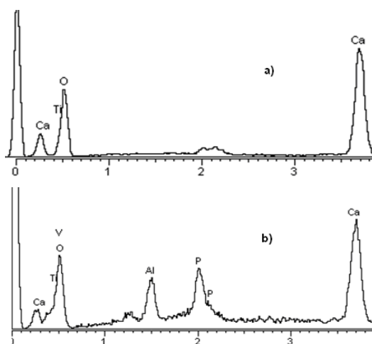
Figura 2. Espectros de EDS para deposiciones a a) 25°C y b) 60°C.
