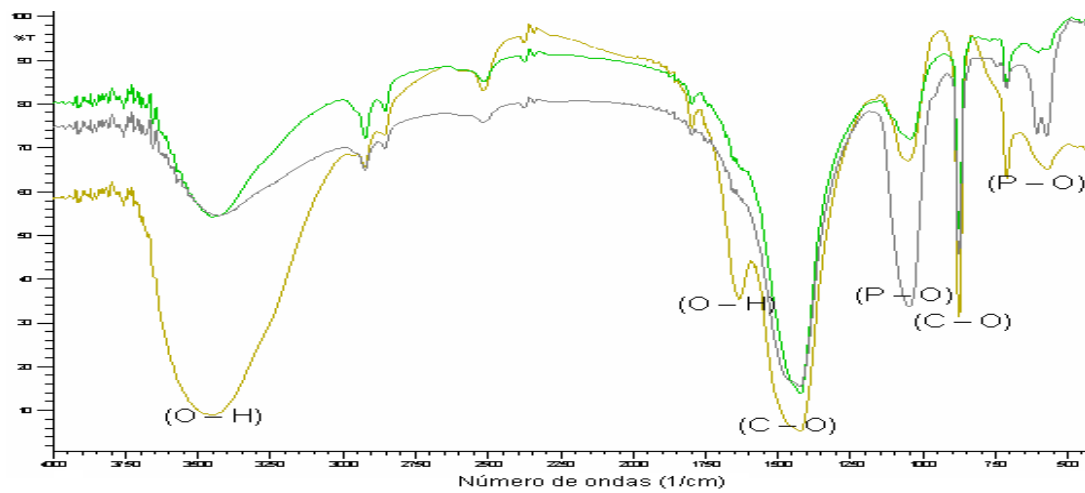
Figura 4. Espectros de infrarrojo para recubrimientos a 25 °C (amarillo y verde) y a 60 °C (gris).
