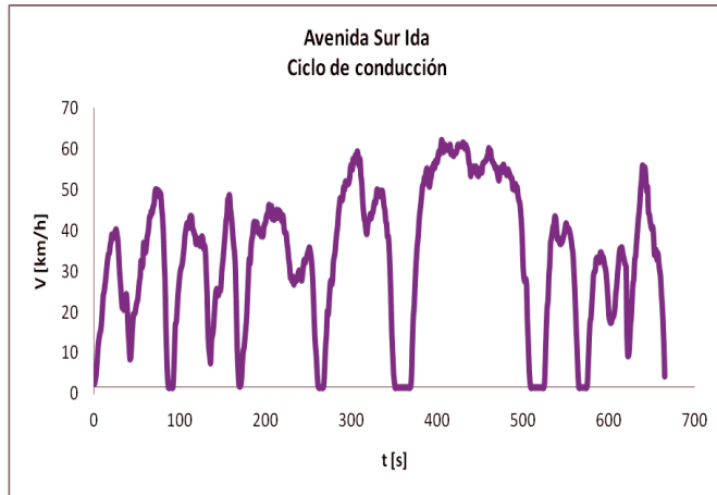
Figura 4. Ciclo de conducción representativo para la ciudad de Pereira
