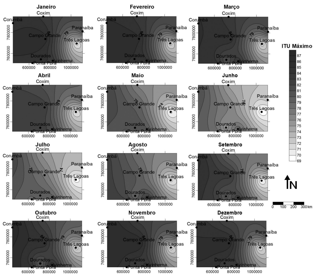
Figura Nº 3 Distribuição espacial e temporal do índice máximo de temperatura e umidade mensal (ITUmáx), para o estado de Mato Grosso do Sul, no período compreendido entre os anos de 1981 e 2008
