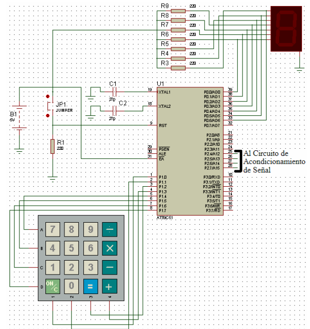
Figura 4. Circuito de control.
