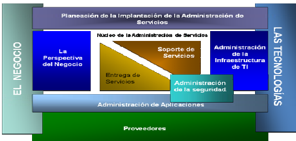
Figura 2. Estructura ITIL
