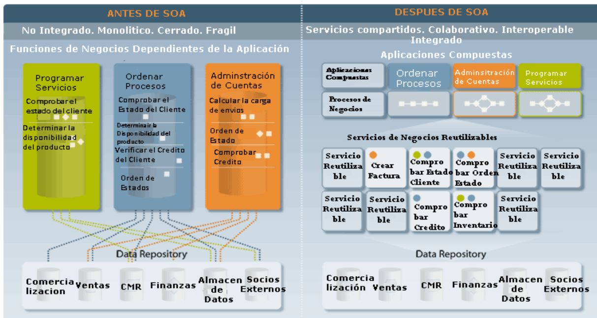
Figura 1. Arquitectura Orientada a Servicios. www.es.sun.com/practice/software/soa . Septiembre-2008
