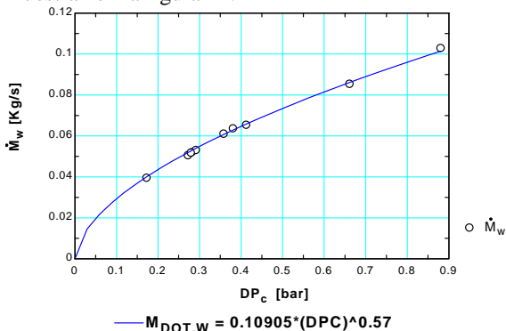
Figura 11. Resultados de ensayos de pérdida de carga.
