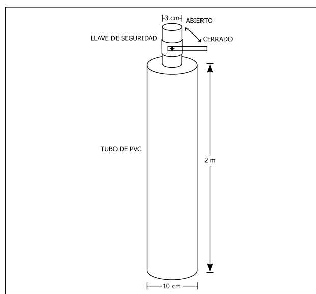
Figura 2. Representación esquemática del tubo de PVC construido para coleccionar las muestras de plancton
