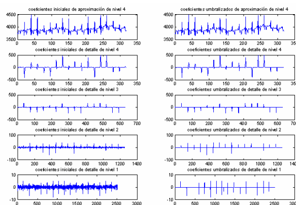
Figura 4. Descomposición y umbralización del registro 100 utilizando una ventana de 13.8 segundos.
