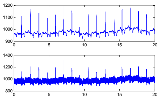
Figura 6. Señal comprimida en el receptor. Reconstrucción wavelet de los coeficientes umbralizados y codificados.
