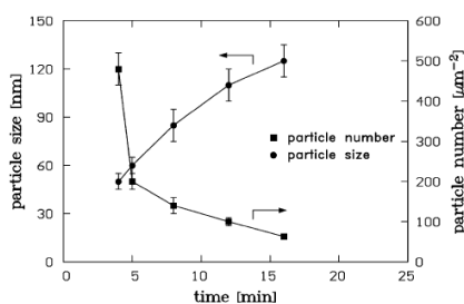
Figura 6 El tamaño de partícula (lado izquierdo) y número de partícula (lado derecho) como función del tiempo de deposición.
