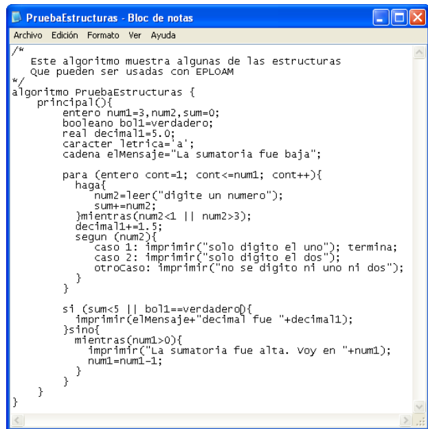
Figura 3. Ejemplo archivo PruebaEstructuras.epl.
