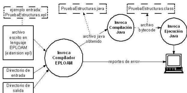
Figura 11. Procesos invocados por el archivo por lotes.
