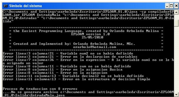
Figura 10. Ejemplo de la salida del procesamiento de un archivo con errores.
