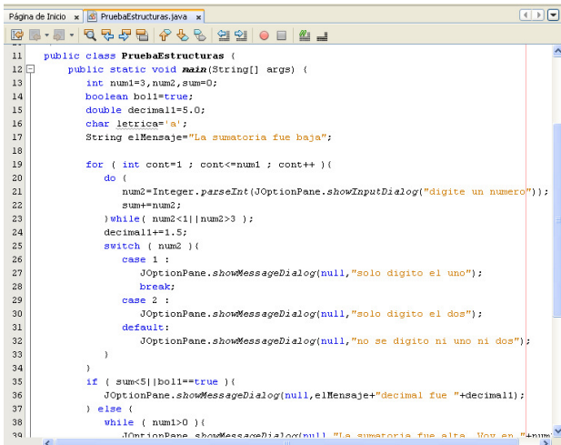
Figura 8. Archivo PruebaEstructuras.java generado por el compilador de EPLOAM abierto en Netbeans.
