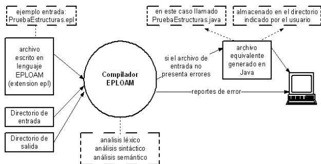
Figura 2. Arquitectura proceso de compilación en EPLOAM.
