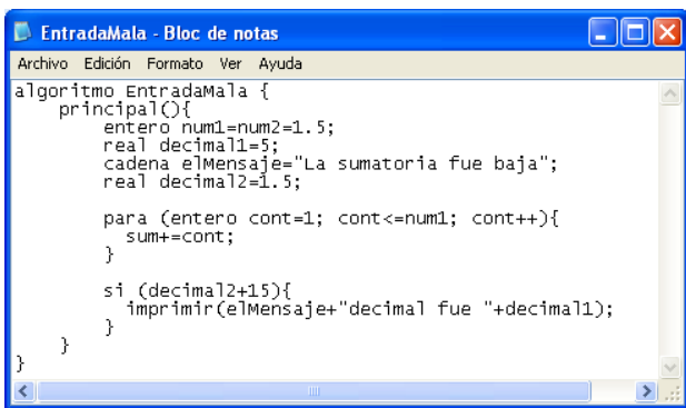
Figura 9. Ejemplo archivo de entrada con errores.
