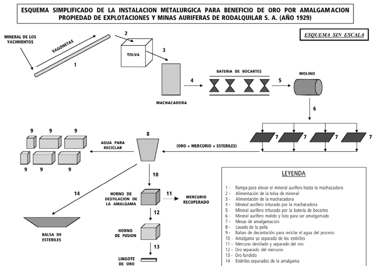
Figura 4. Esquema simplificado del funcionamiento de la instalación metalúrgica aurífera por amalgamación de la empresa Explotaciones y Minas Auríferas de Rodalquilar S.A. (año 1929).
