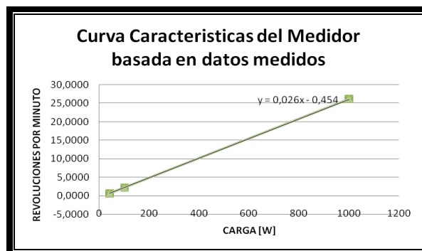
Figura 5. Curva característica del medidor.
