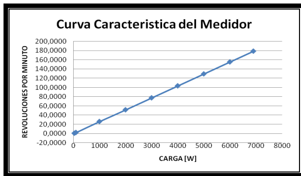
Figura 6. Curva característica del medidor.
