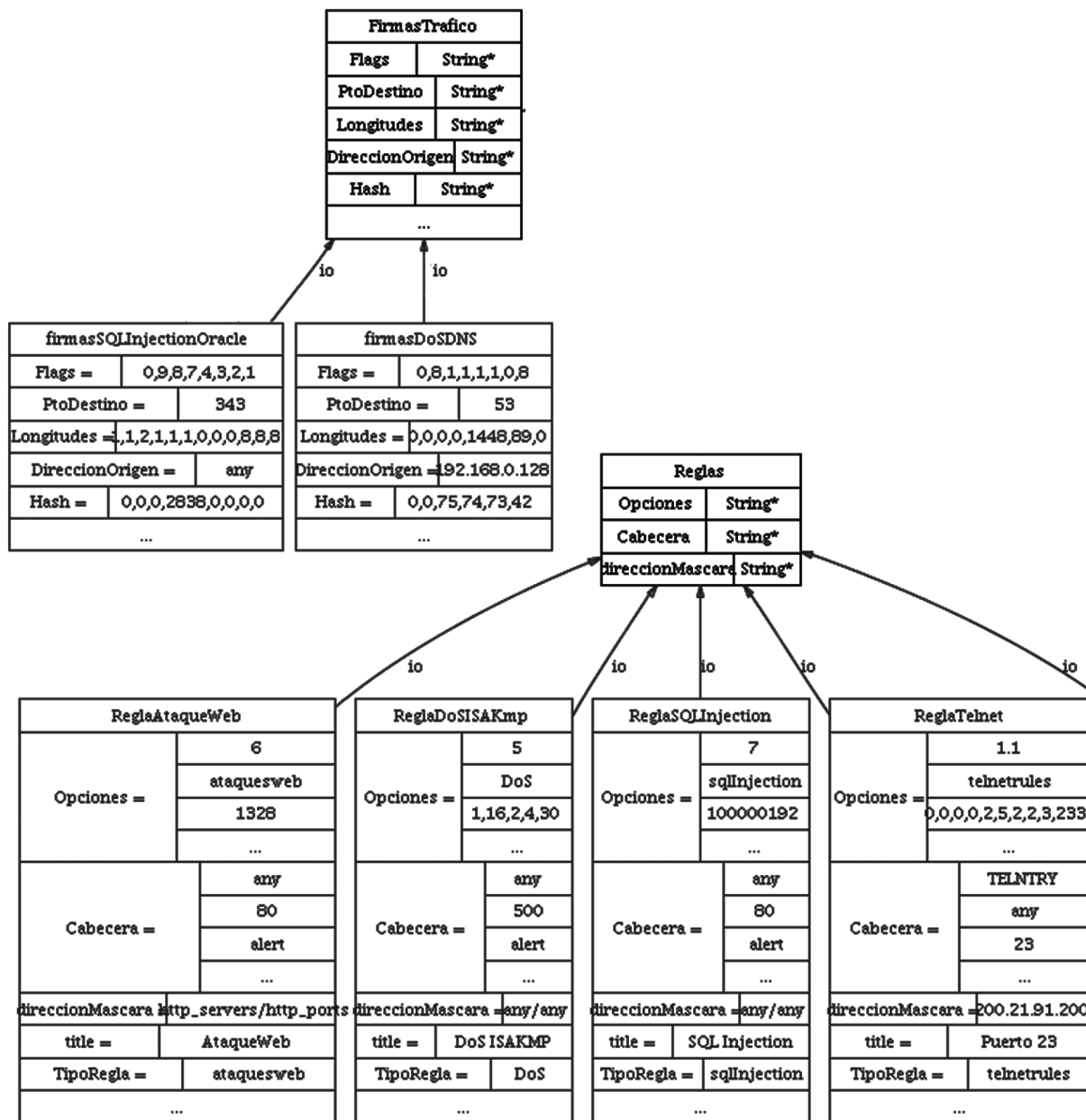
(b) Fragmento de representación ontológica par firmas de inyección SQL, Dos y Acceso Telnet No Autorizado.
