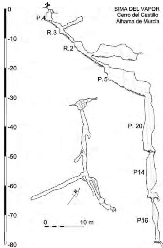
Figura 13. Plano de la Sima del Vapor.
