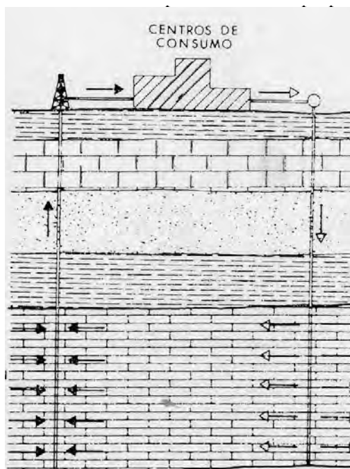
Figura 16. Sistema de aprovechamiento propuesto.
