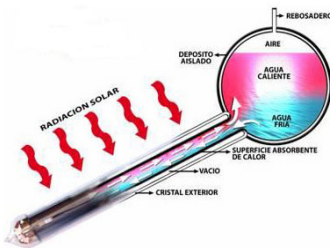
Figura 7. Transferencia de calor por efecto termosifón en tubos de vacío. [9]
