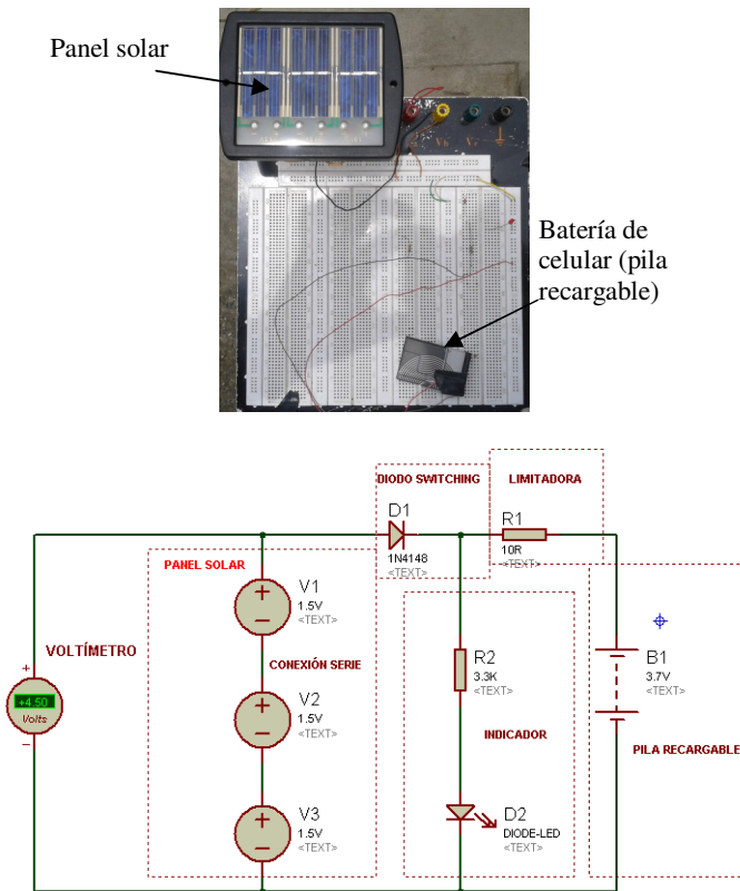
Figura 10. Cargador solar y circuito de conexión
