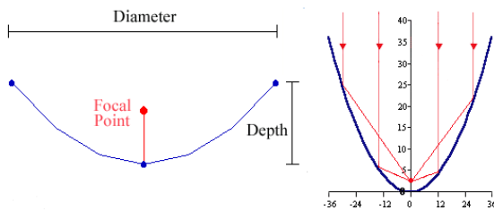
Figura 2. Diseño parabólico de cocina
