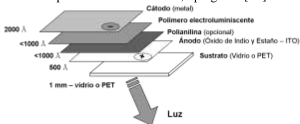
Figura 7. Estructura de un dispositivo PLED fabricado con polímeros semiconductores.
