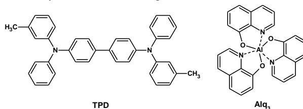
Figura 6. Moléculas orgánicas pequeñas empleadas en el primer SMOLED reportado en la literatura.
