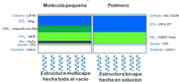
Figura 5. Estructuras de capas para un SMOLED y un PLED . NPB: N,N -di(naftalen-1-il)- N,N' -difenilbencidina; CuPc: ftalocianina de cobre; PPV: polifenilenvinileno; PF: polifluoreno; PDOT: poli(dioctilbitiofeno); pani: polianilina.
