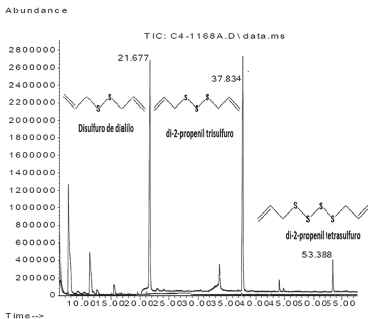
Figura 1. Compuestos del grupo de sulfuros resultantes de la degradación de la aliina presentes en la oleorresina de ajo identificados por GC-MS obtenida del cromatógrafo de gases 6890N con detector selectivo de masas 5973 Network.
