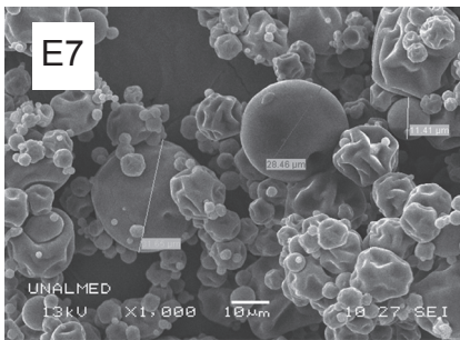
Figura 3. Fotografías SEM de las microcápsulas de las muestras E1, E2, E3, E5, E6, E7 y E8.
