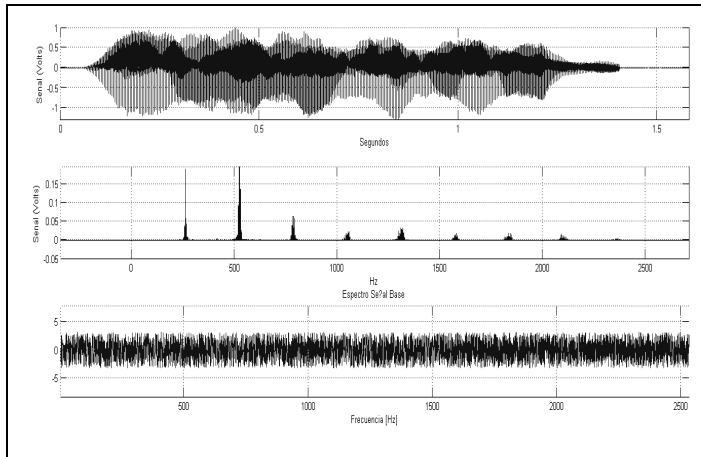
Figura 9. Forma de onda y espectro en amplitud y fase para la flauta en Do central.
