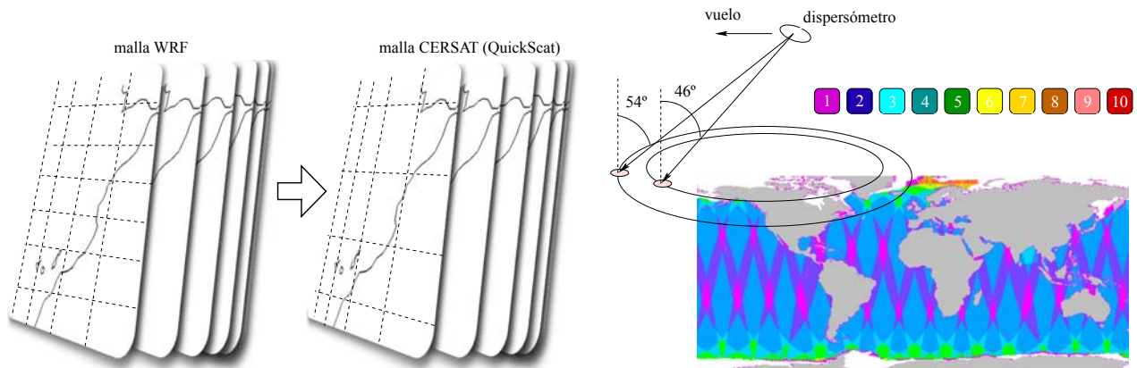
Figura 9. Mallado espacial utilizado para la correlación entre los vientos predichos por el WRF y los obtenidos a partir de los datos generados por el satélite QuickScat (izquierda). Funcionamiento general y número de pasadas del dispersómetro SeaWinds (derecha)
