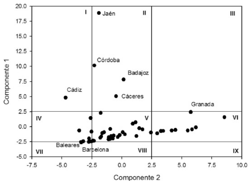
Figura 2. Diagrama de componentes principales para las variables anuales de desempleo y superficie repoblada de cada una de las provincias
