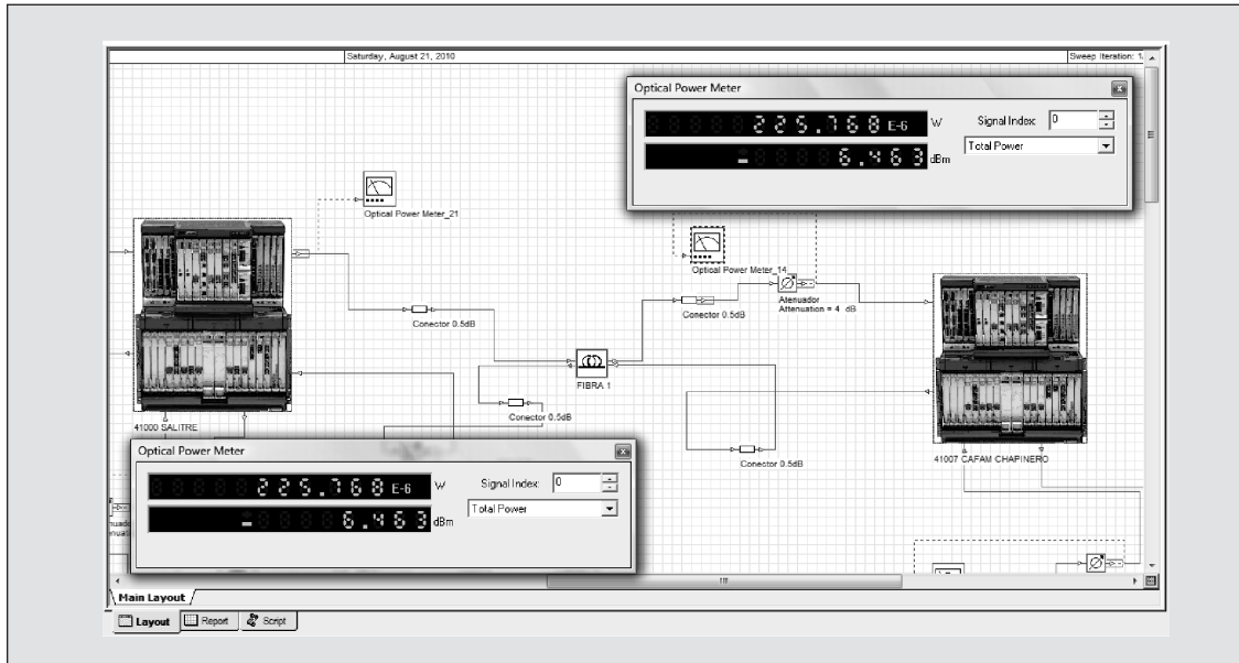
Figura 9. Resultados de medición 2: Potencia de recepción con atenuador.
