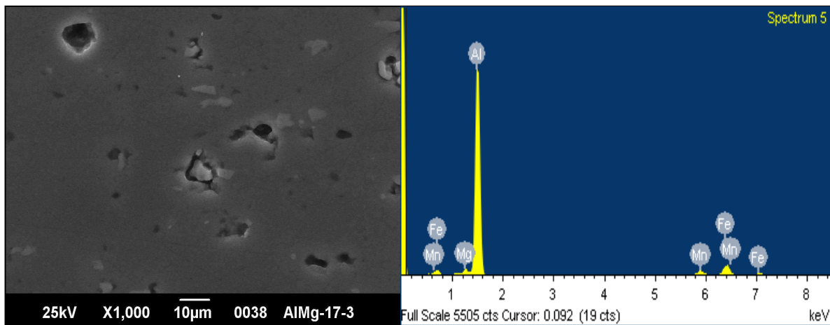
FIGURA 4. Micrografía electrónica de precipitados (Fe,Mg,Mn)Al en la soldadura
