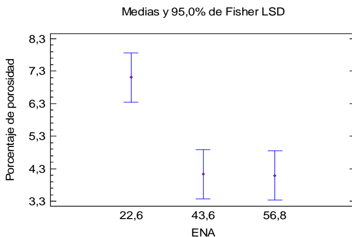
FIGURA 5. Gráfica de Medias de Varianza con 95,0 % de confiabilidad de Fisher
