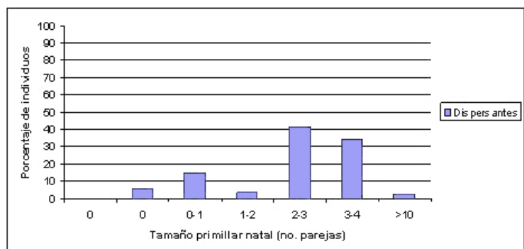
Figura 7. Porcentaje de individuos dispersantes desde cada primillar según el tamaño de la colonia de origen (en número de parejas).
