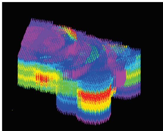
Figura 2. Modelo de bloques. Fuente: MineSight®
