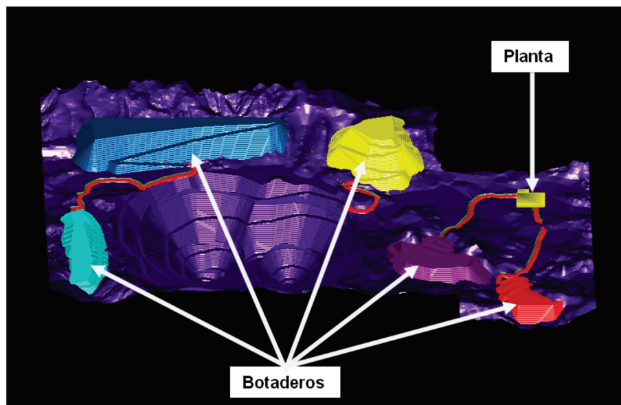
Figura 4. Pit final con disposición de botaderos y planta de beneficio Fuente: MineSight®
