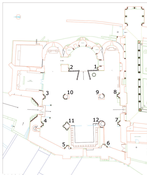
Figura 3: Planta con la numeración de los soportes.
