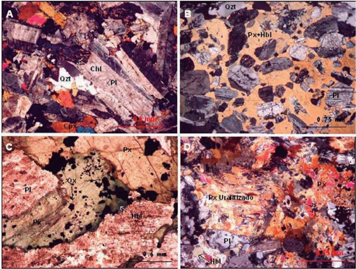
FIGURA 2. A. Hábito tabular de las plagioclasas (Pl) con pequeños intersticios rellenos por clinopiroxenos (Cpx), algunos reemplazados pseudomórficamente por clorita (Chl). B. Textura Ofítica de plagioclasas en Piroxeno alterado a Hornblenda (Px+Hbl). C. alta concentración de Óxidos de Fe-Ti en el líquido intercúmulo (Ox), que a su vez el cambio de color indica la transformación Piroxeno a Hornblenda. D. Uralitización intensa en los piroxenos
