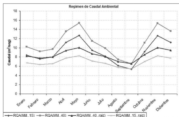
Fig. 3. Régimen de caudal con MM 40 y MM 15 Estación Limnigráfica Mateguadua - periodo: 1975-1995.
