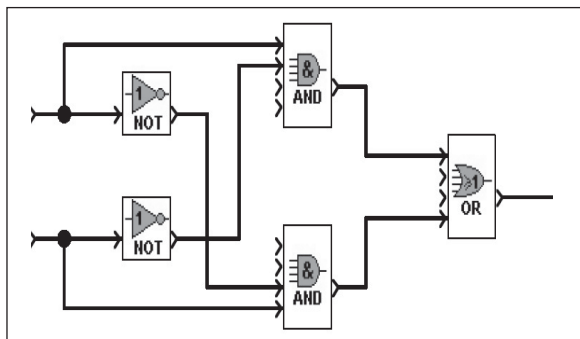
Fig. 2. Ejemplo de diseño por bloques funcionales.
