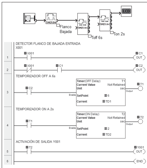
Fig. 3. Traducción bloques funcionales a diagrama ladder
