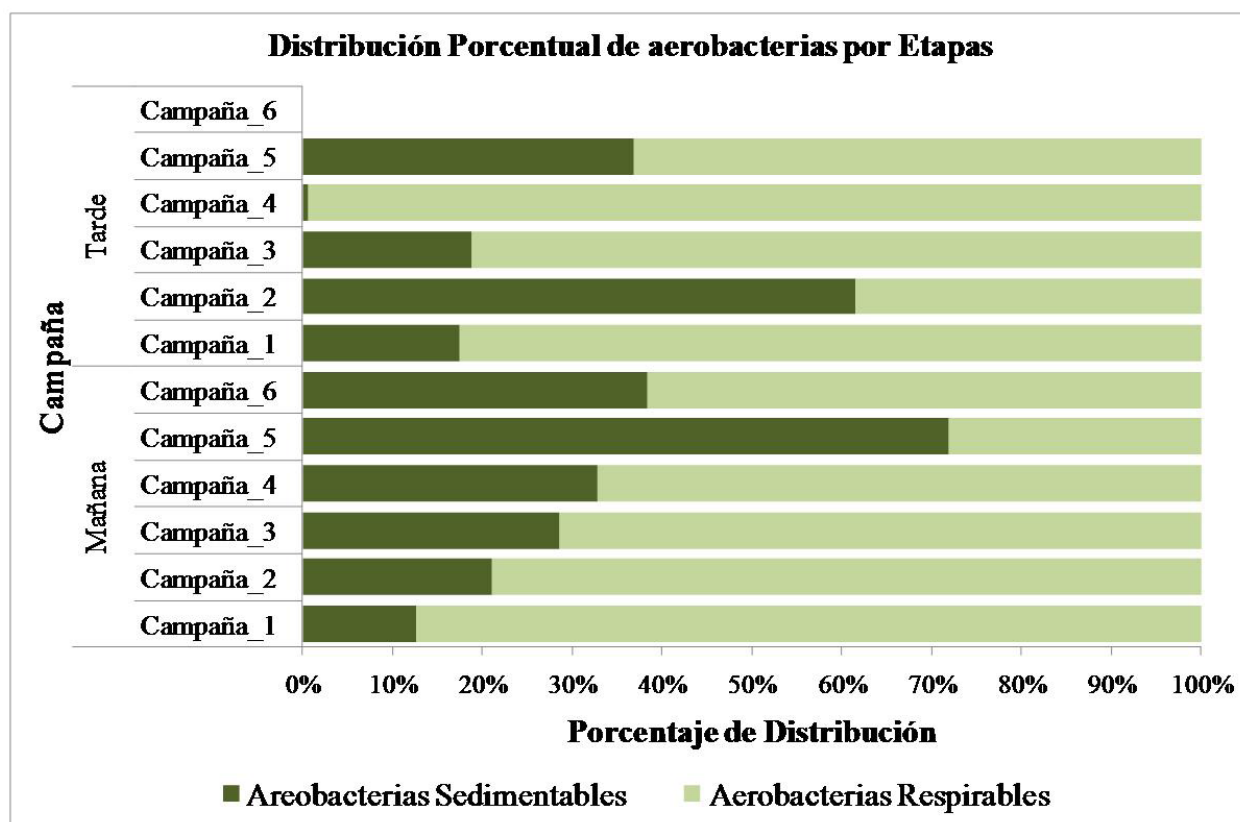
Figura 2. Distribución porcentual de los diámetros de las aerobacterias
