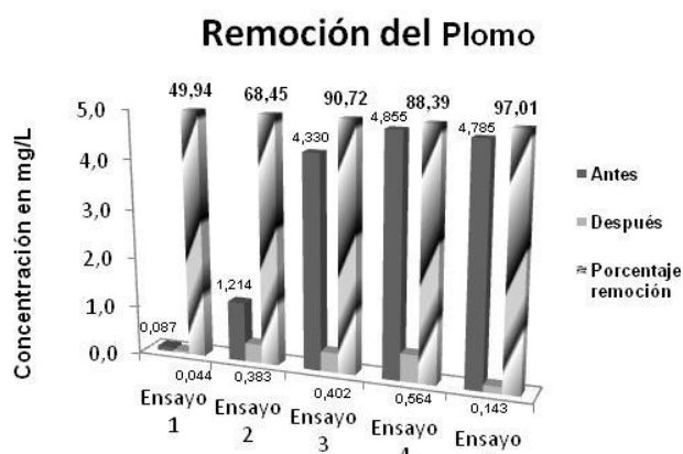
Figura 4. Eficiencia de la batería de filtros en la remoción del plomo
