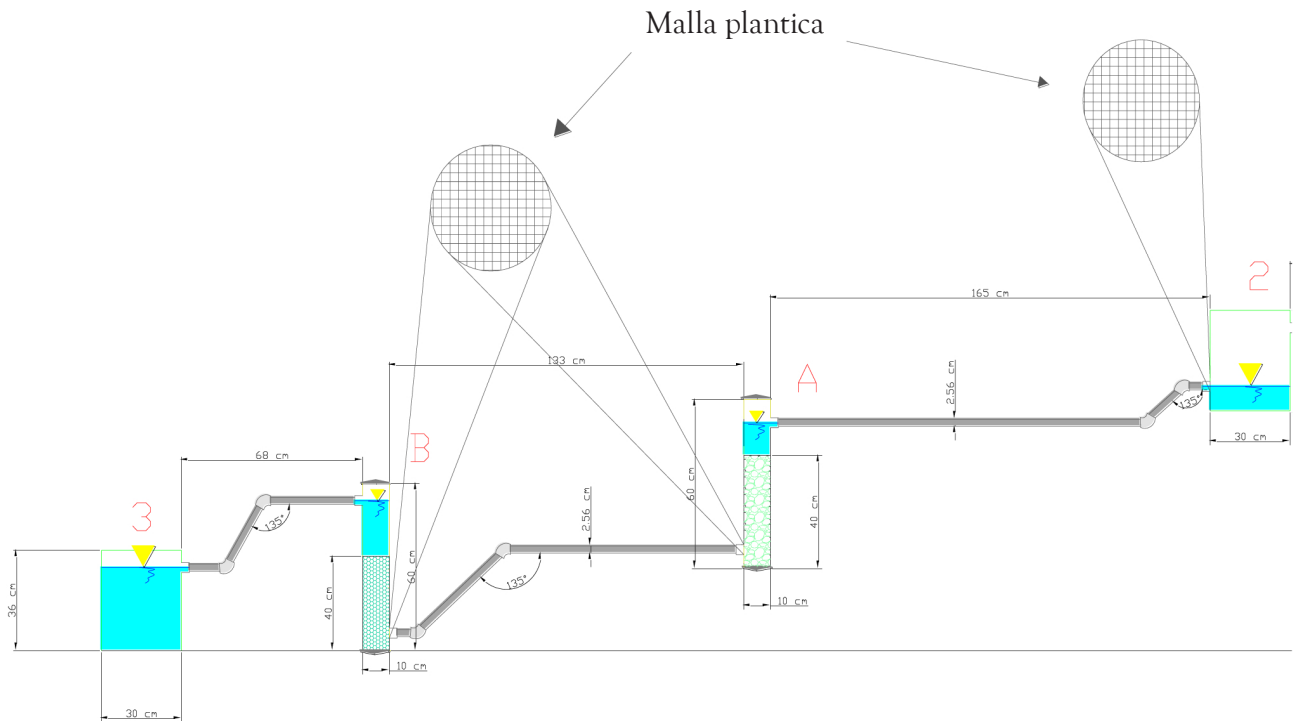
Figura 2. Detalle diseño batería de filtros
