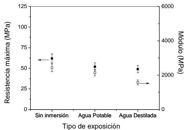
Fig. 3. Comportamiento a flexión de composites con fibras sin tratar sometidas a diferentes tipos de exposición
