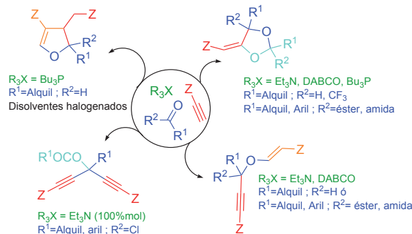
Figura 3. Procesos dominó basados en la generación organocatalítica de aniones acetiluro en presencia de compuestos carbonílicos.
