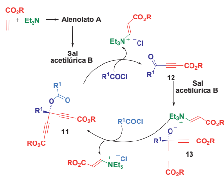
Esquema 6. Síntesis \text{A}_2\text{BB}' 4CR de diinos alternados 11.
