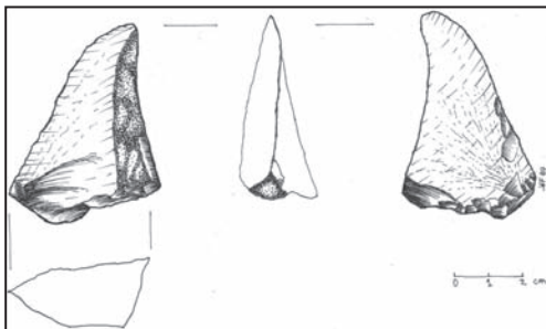
Figura 7. FNRC en metagrauvasca (artefacto número 1 de la Tabla 1).
