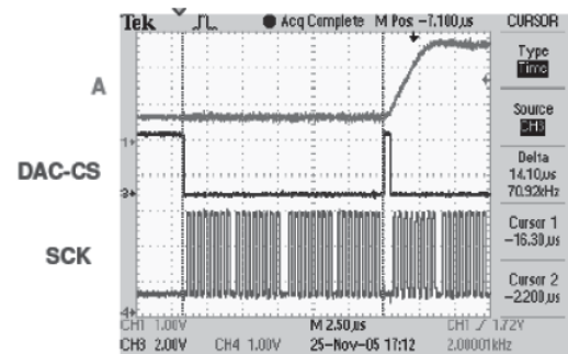
Figura 20. Conversión análoga digital.
