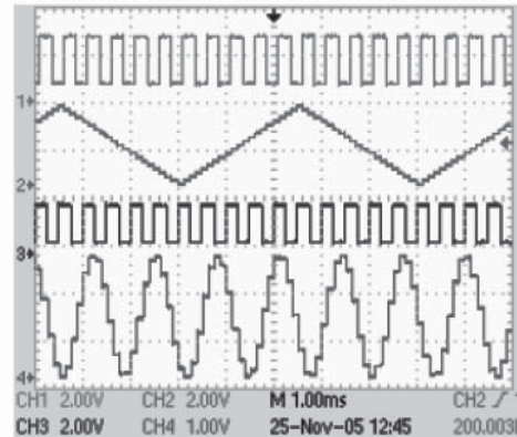
Figura 19. Muestreo de varias señales a la salida de los canales de conversión.
