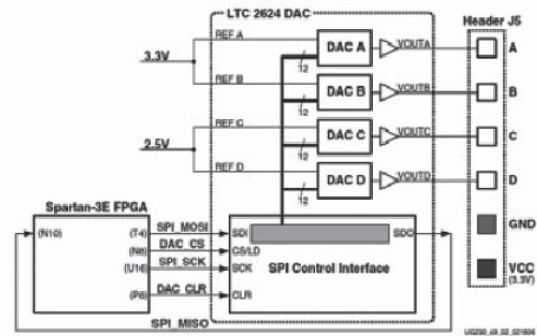
Figura 13. Interfaz salida de conversión digital-análogo [2].
