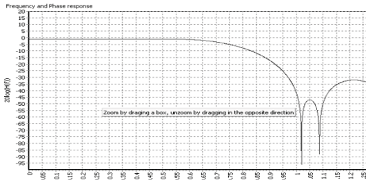
Figura 12. Respuesta en frecuencia pasa bajo.
