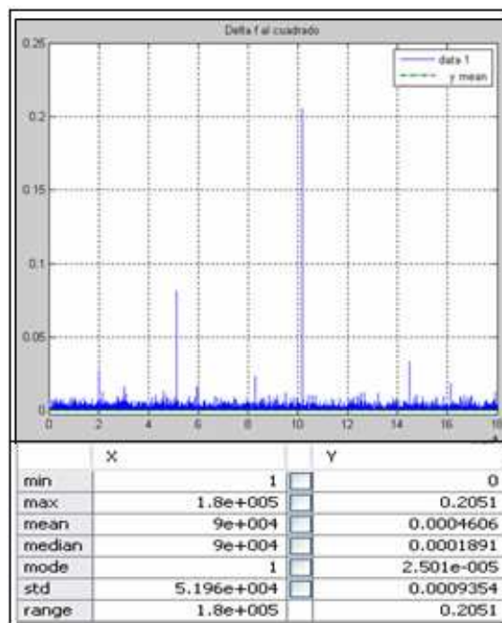
Fig. 2.3.1. Valores de las desviaciones de la frecuencia elevados al cuadrado.
