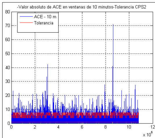
Fig.3.2.1.Verificación CPS-2 para \epsilon_{10} = 11.5 mHz.
