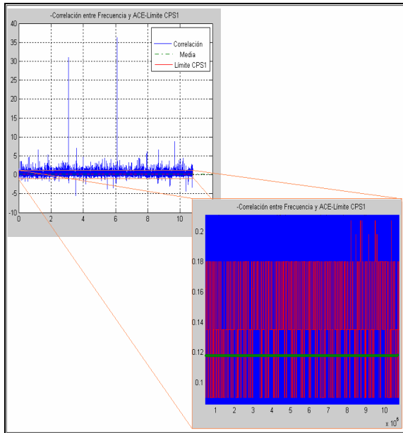
Fig. 3.1.1 (b). Verificación CPS-1 con \epsilon_1= 30\text{mHz} .
