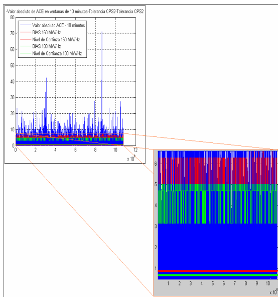
Fig. 3.2.2. rendimiento del control secundario aumentando el valor mínimo del BIAS asignado en el sistema eléctrico del Ecuador.
