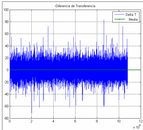
Fig.3.1 (b).Desviaciones de la Transferencia.
