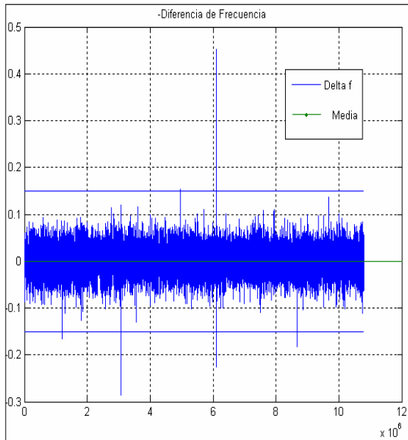
Fig. 3.1(a).Desviaciones de la Frecuencia.
