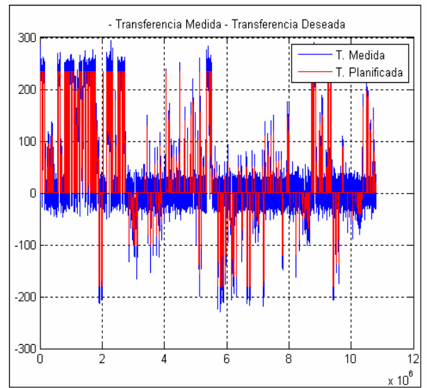
Fig. 3.1(c). Transferencia Mediada Vs. Transferencia Planificada.
