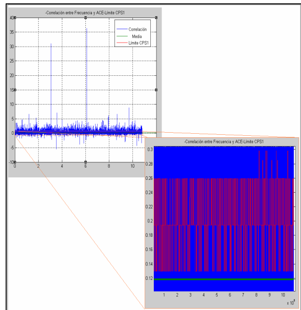
Fig. 3.1.1 (a).Verificación CPS-1 con \epsilon_1= 36\text{mHz} .
