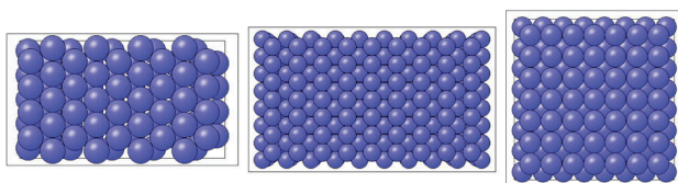
Figura 2. Representación esquemática de los planos de base de un cristal cúbico centrado en las caras. De izquierda a derecha: Pt(111), Pt(110), Pt(100).
