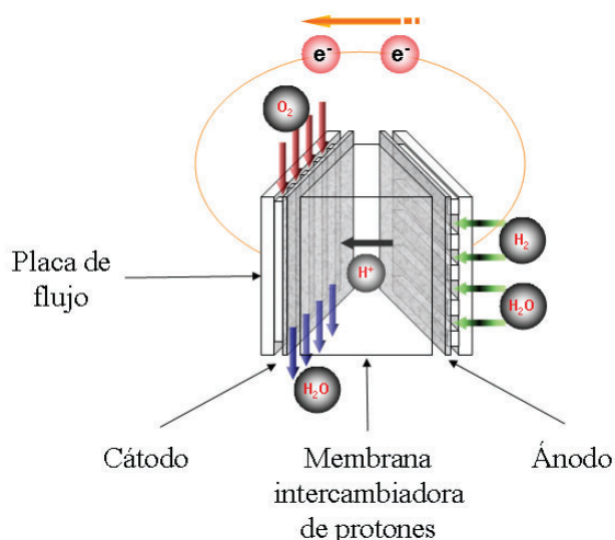
Figura 1. Funcionamiento y componentes de una celda de combustible de electrolito polimérico sólido.
