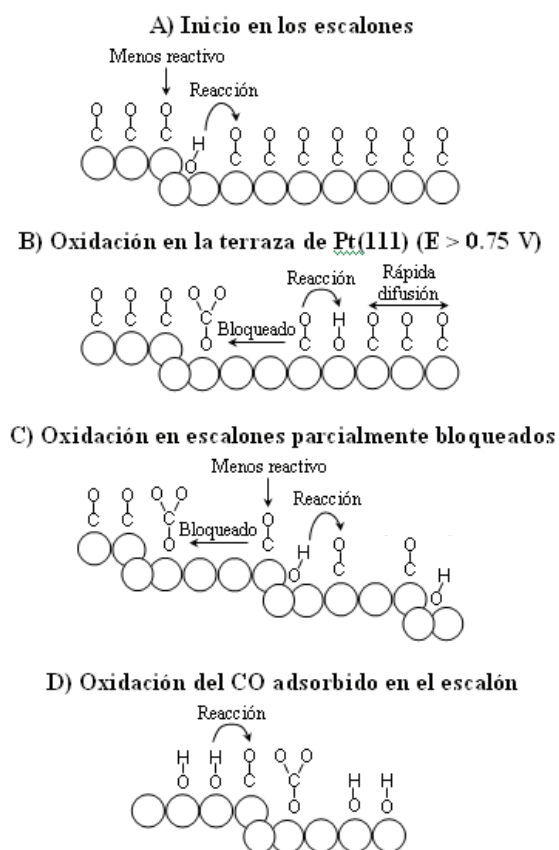
Figura 9. Representación esquemática del mecanismo de oxidación de CO sobre superficies escalonadas de Pt en medio alcalino.
