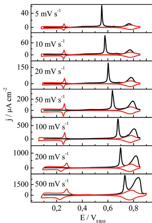
Figura 7. Oxidación voltamperométrica de \text{CO}_{\text{ad}} (línea negra) y el siguiente voltamperograma cíclico (línea roja) sobre Pt(554) en NaOH 0,1 M a distintas velocidades de barrido de potencial. E_{\text{ad}} = 0,1 \text{ V} . Reproducido con permiso de Elsevier ref. [38]
