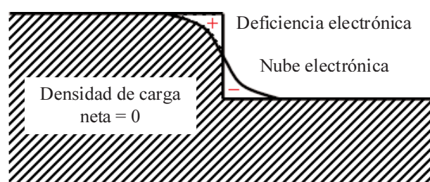
Figura 4. Representación esquemática de la distribución de la densidad de carga en una superficie escalonada.
