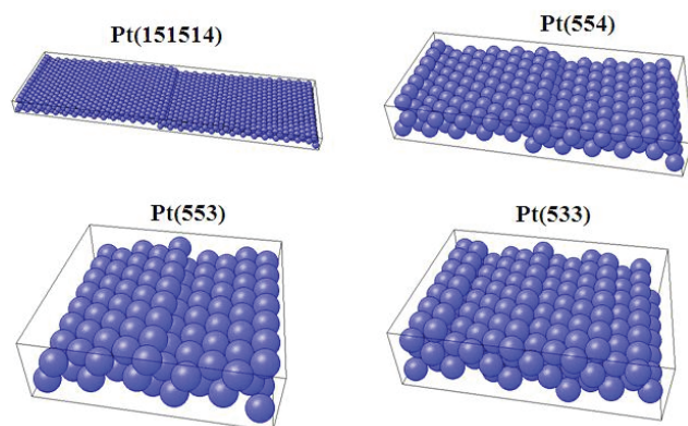
Figura 6. Representación esquemática de las superficies escalonadas observadas en la Figura 5.
