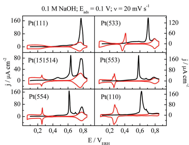
Figura 5. Oxidación voltamperométrica de CO ad (línea negra) y el siguiente voltamperograma cíclico (línea roja) sobre Pt(111), Pt(151514), Pt(554), Pt(553), Pt(533) y Pt(110) en NaOH 0,1 M. v = 20 \text{ mV s}^{-1} . E_{\text{ad}} = 0,1 \text{ V} . Reproducido con permiso de la ref.[38]
