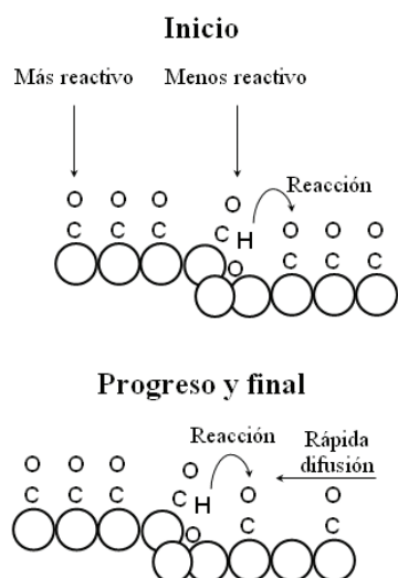
Figura 8. Representación esquemática del mecanismo de oxidación de CO sobre superficies escalonadas de Pt en medio ácido.
