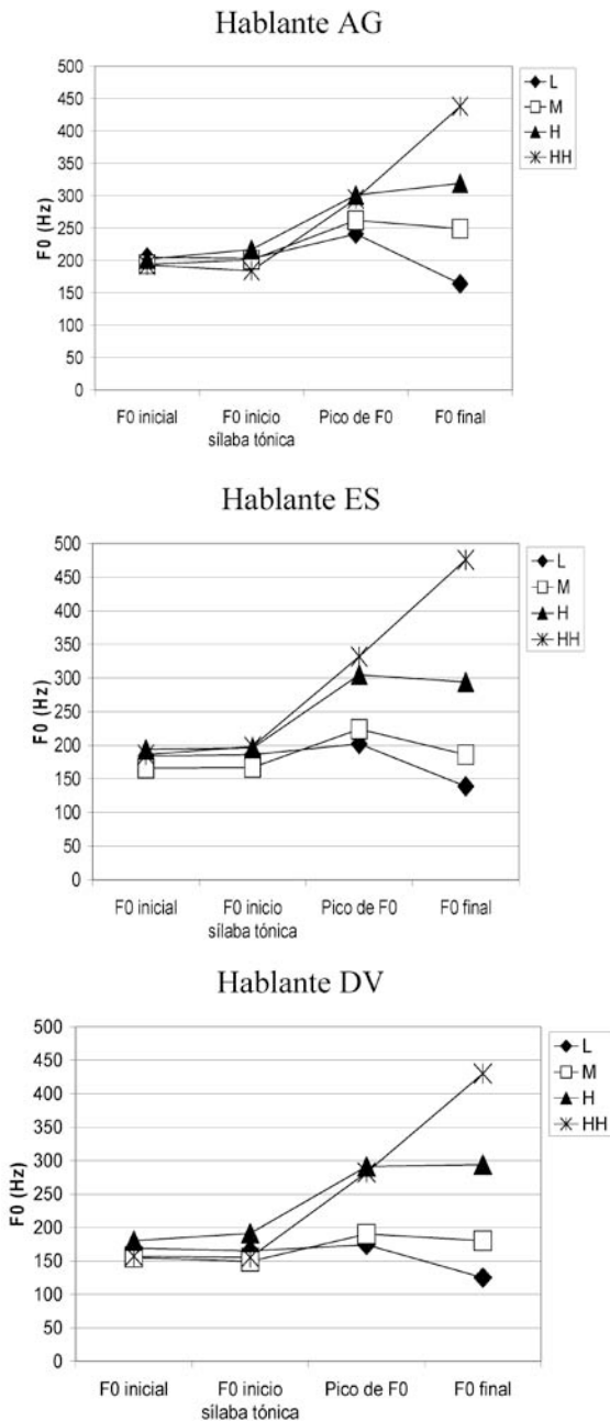
FIGURA 7 Esquematización de las curvas de F0 de las tres informantes a partir de las medias obtenidas de los valores de F0
