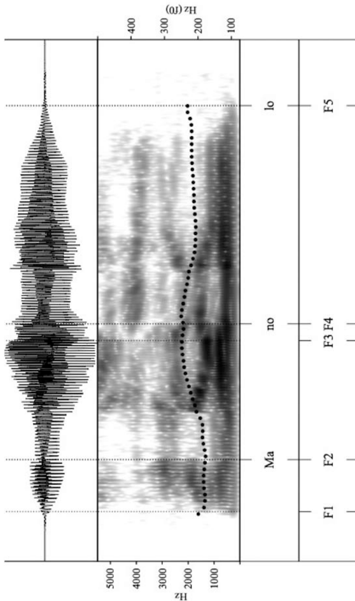
FIGURA 5 Oscilograma, espectrograma y curva de FO, fronteras silábicas y valores de FO para el enunciado Ma n o l o producido como enumeración inacabada por la informante AG
