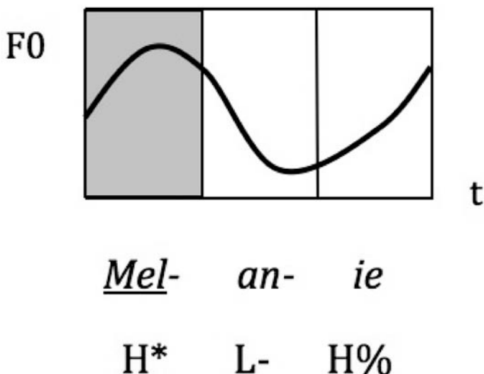
FIGURA 2 Esquematación y modelización de un contorno de FO descendente-ascendente en la palabra Melanie mediante el modelo MA
