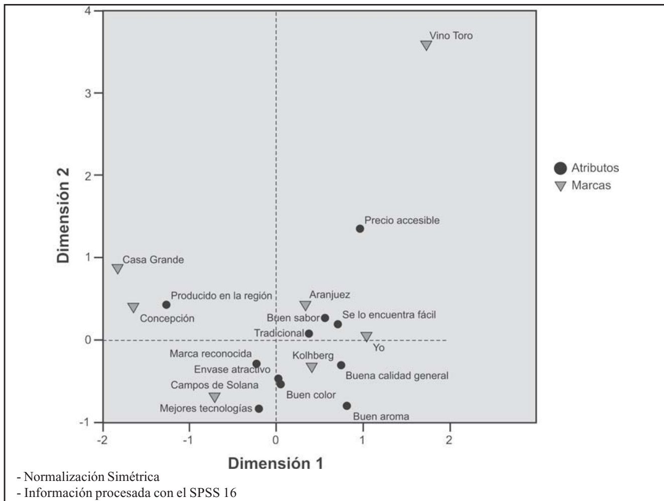
Figura 3 Mapa Perceptual. Puntos columna y fila
