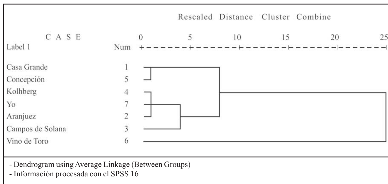
Figura 4 Dendograma Análisis Cluster Jerárquico
