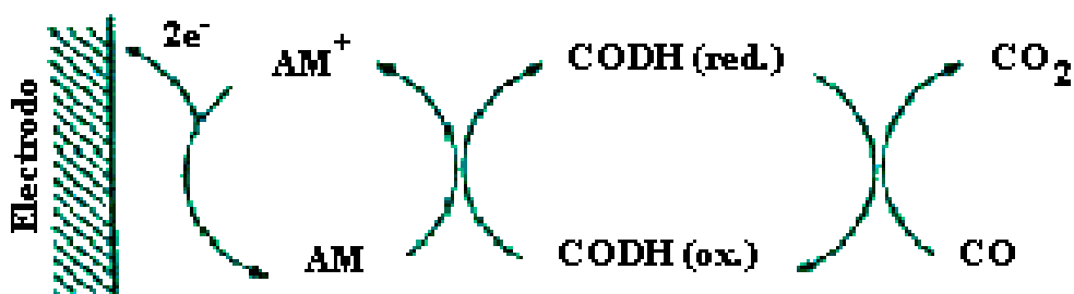
Oxidación electroquímica de monóxido de carbono con el uso de azul de metileno (AM + ) como un mediador electrónico, CODH (red.) y CODH (ox.).
