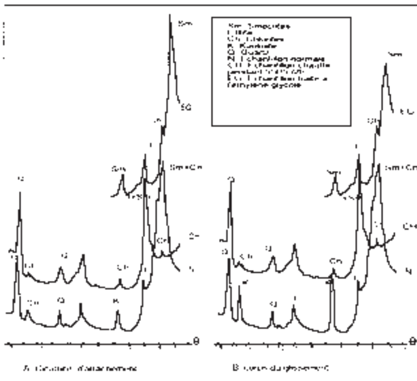
FIGURE 3. Diffractogramme de la fraction fine <10 \mu\text{m} du glissement de Sehb Nejoum.
