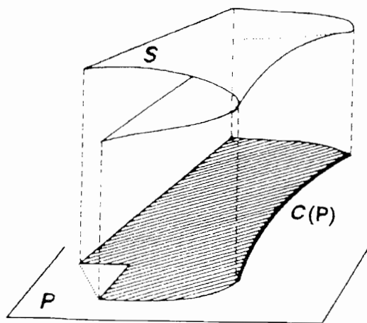
Figura 4 - Projeção de uma superfície S em um plano P. A curva C(P) representa a projeção da dobra de S. A área do triângulo definido pela linha pontilhada descrita em P soma-se à projeção hachurada de S para representar uma das possíveis superfícies de intercepto de S. Modificado de Jacobi & Langevin (1996).
