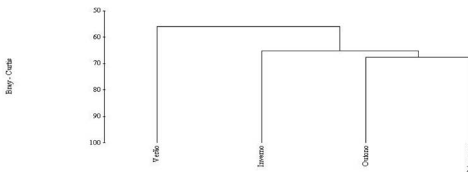
Figura 2. Análise de grupamento das quatro estações do ano, quanto à freqüência das espécies epífitas em Sargassum vulgare da Praia das Gordas, Angra dos Reis, RJ. Coeficiente de similaridade de Bray-Curtis aplicado aos dados não transformados, pelo método de associação média (UPGMA).
