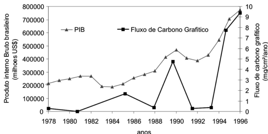
Figura 13. Fluxo de carbono grafítico e o Produto Interno Brasileiro.
